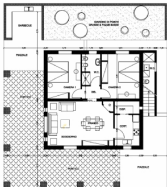
PIANTA PIANO TERRA VILLETTA 2
